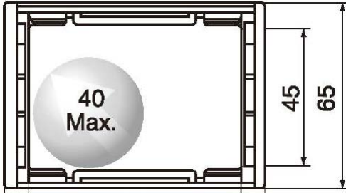
■ 仕切板断面寸法
